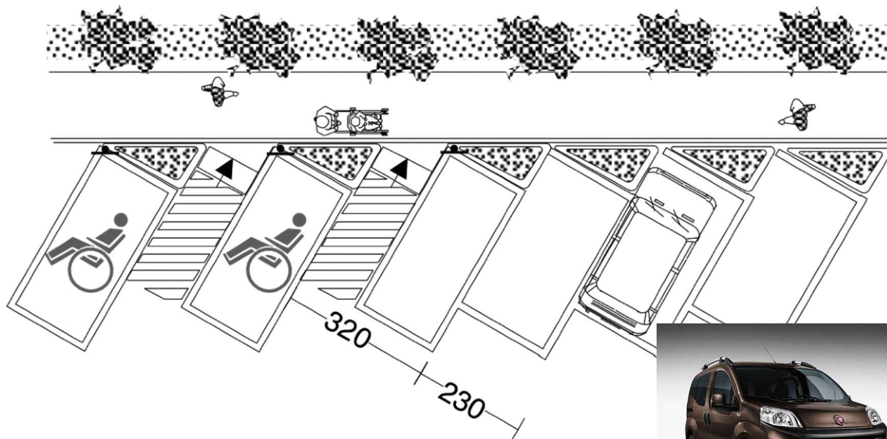
Disposizione a spina di pesce semplice
